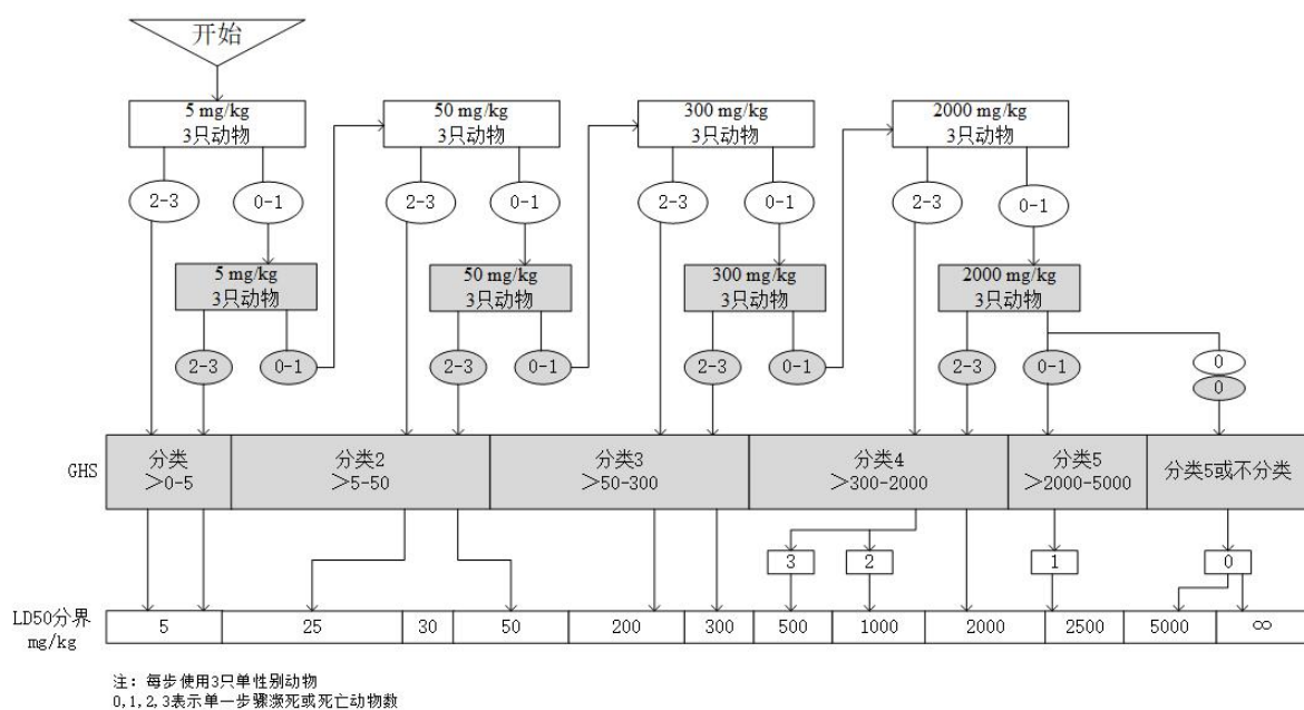
图 1 初始剂量 5 mg/kg 的试验程序
