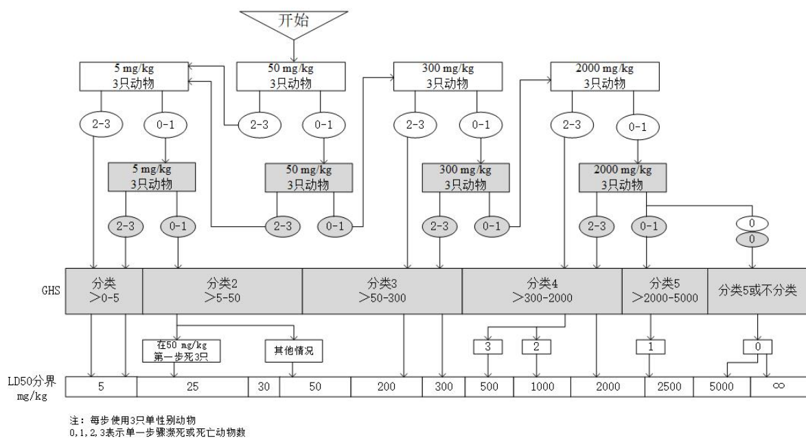
图 2 初始剂量 50 mg/kg 的试验程序
