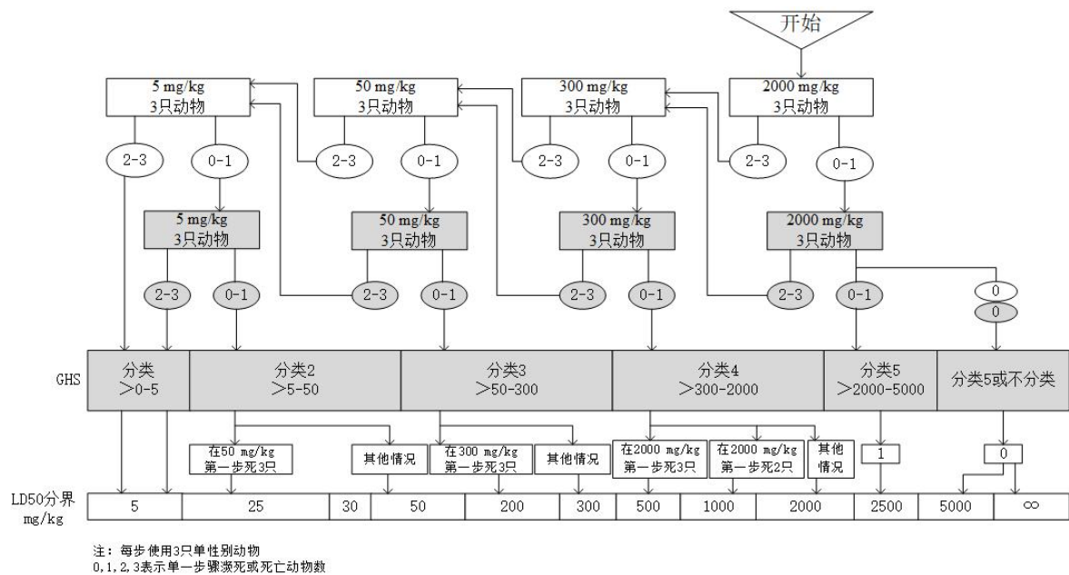
图 4 初始剂量 2000 mg/kg 的试验程序
