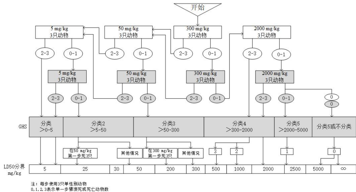
图 3 初始剂量 300 mg/kg 的试验程序
